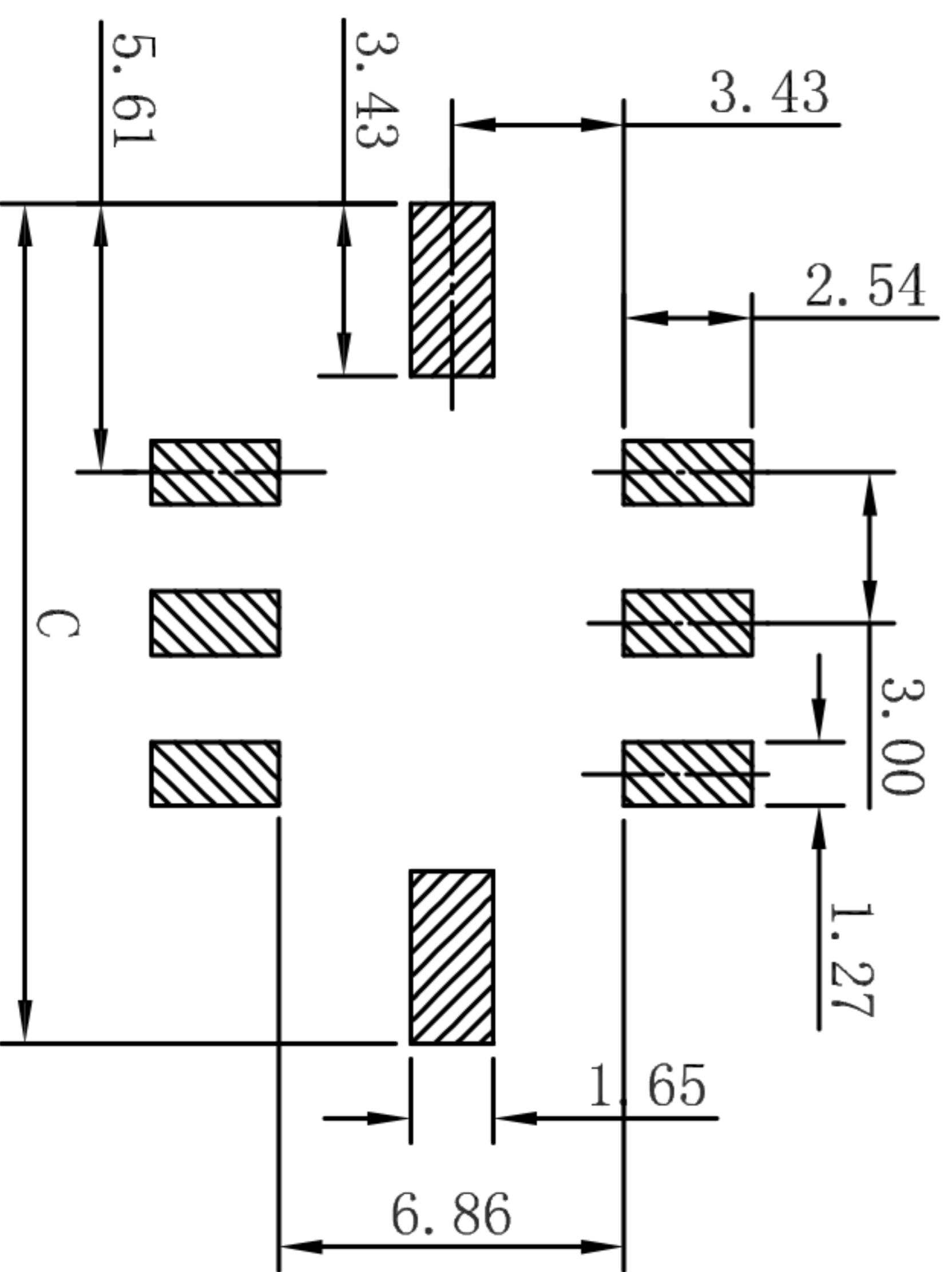
P. C. B. LAYOUT
