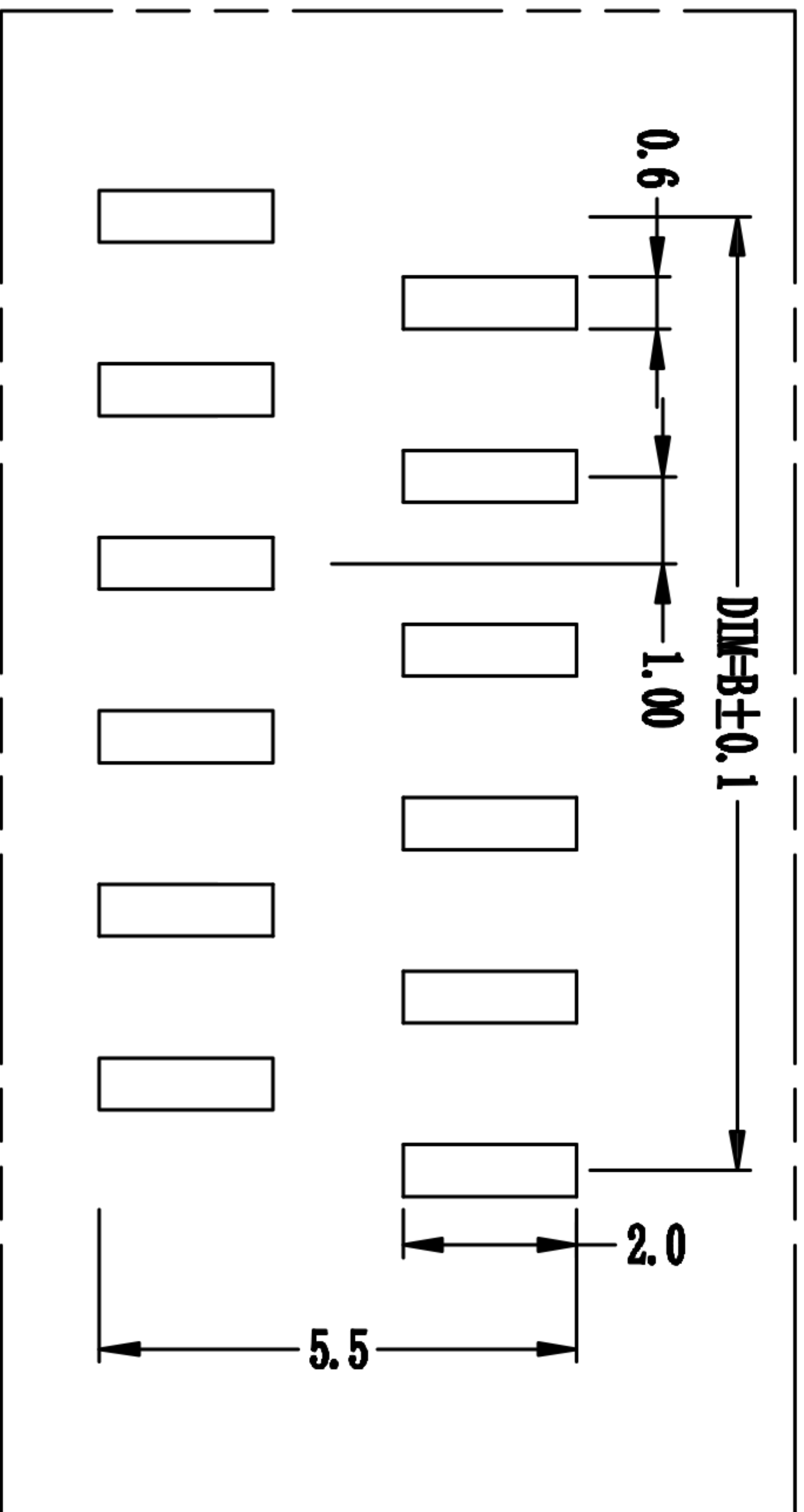
PCB Layout 正脚
