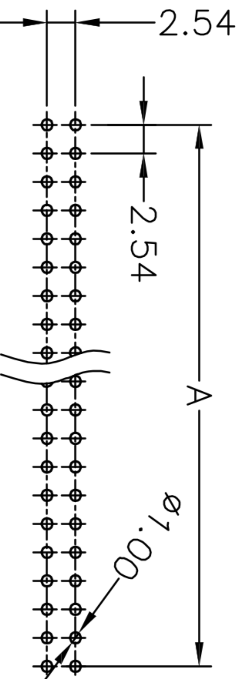
P.C.B. LAYOUT
